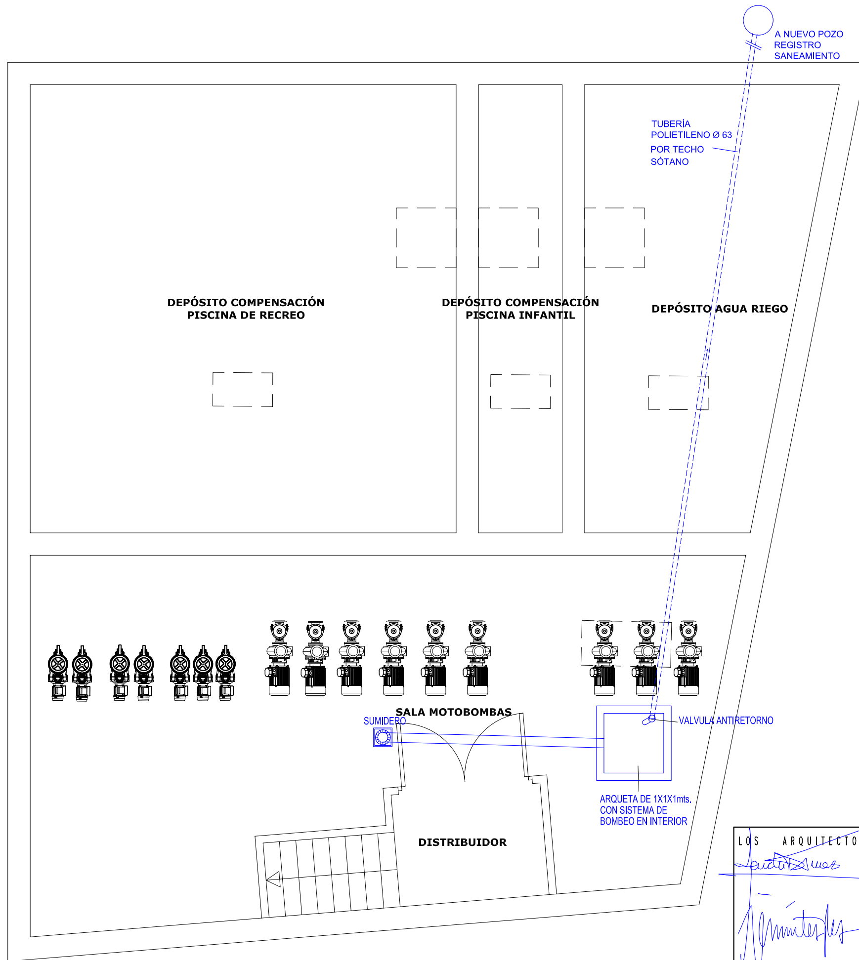
PLANTA SÓTANO
