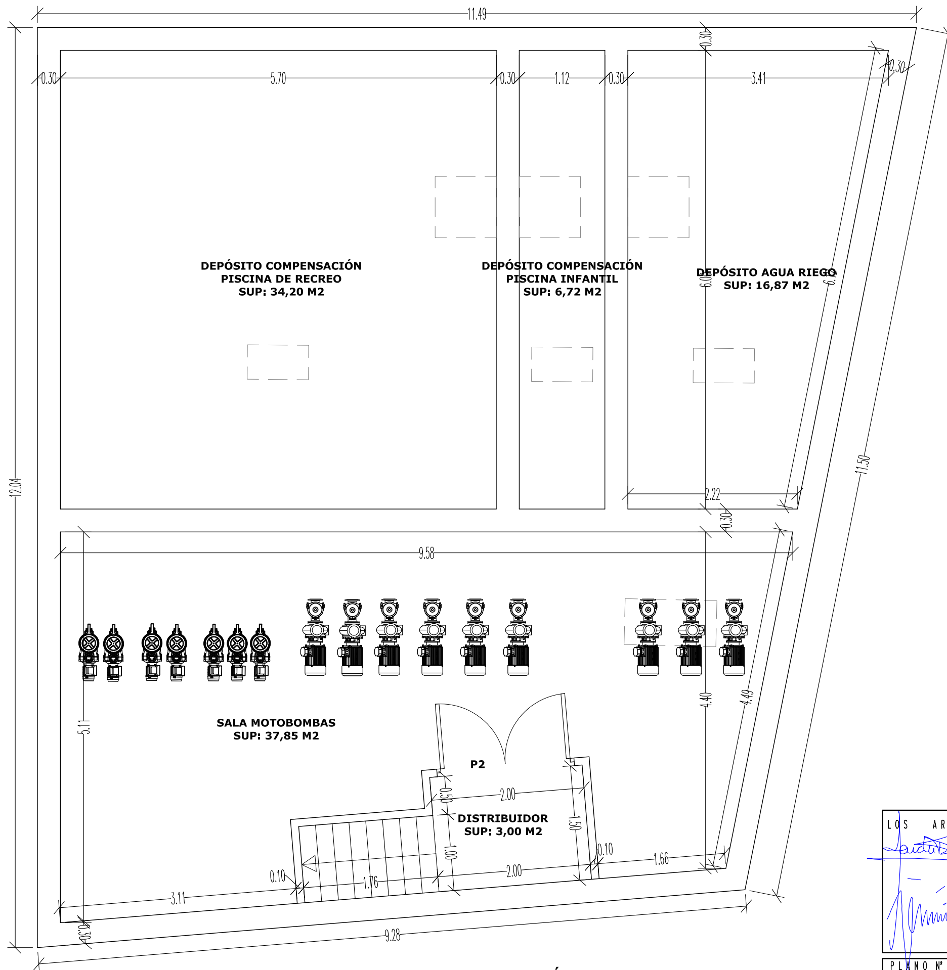
PLANTA SÓTANO
